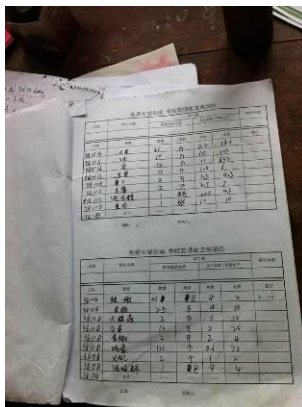
图 14 流水账
