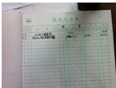
图 15 总账
