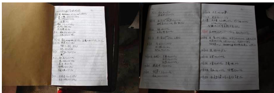
图 13 入库登记
