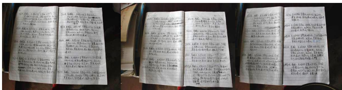
图 14 出库登记
