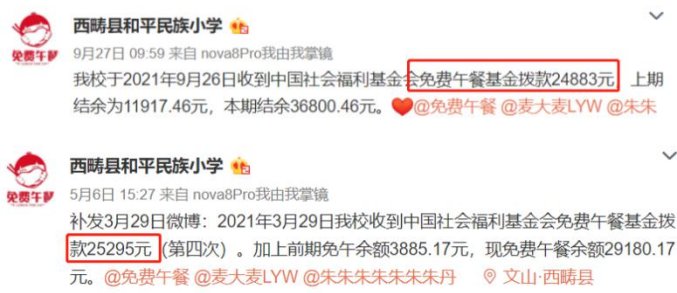
图 2 拨款公示截图
