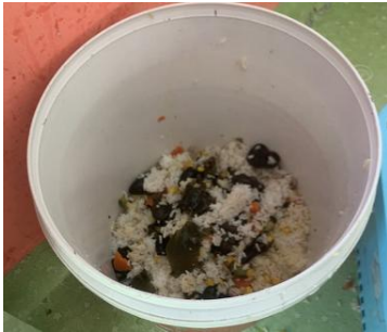
图III-4 餐后倾倒图
